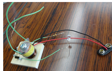
サーチコイルと ドライブコイル
